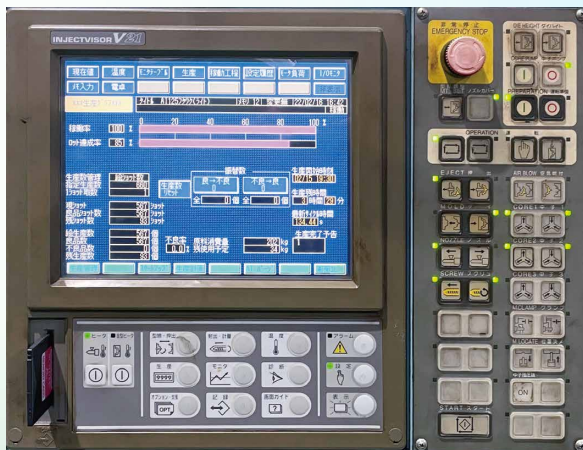
IV-V21 外観(縦型操作パネル)
