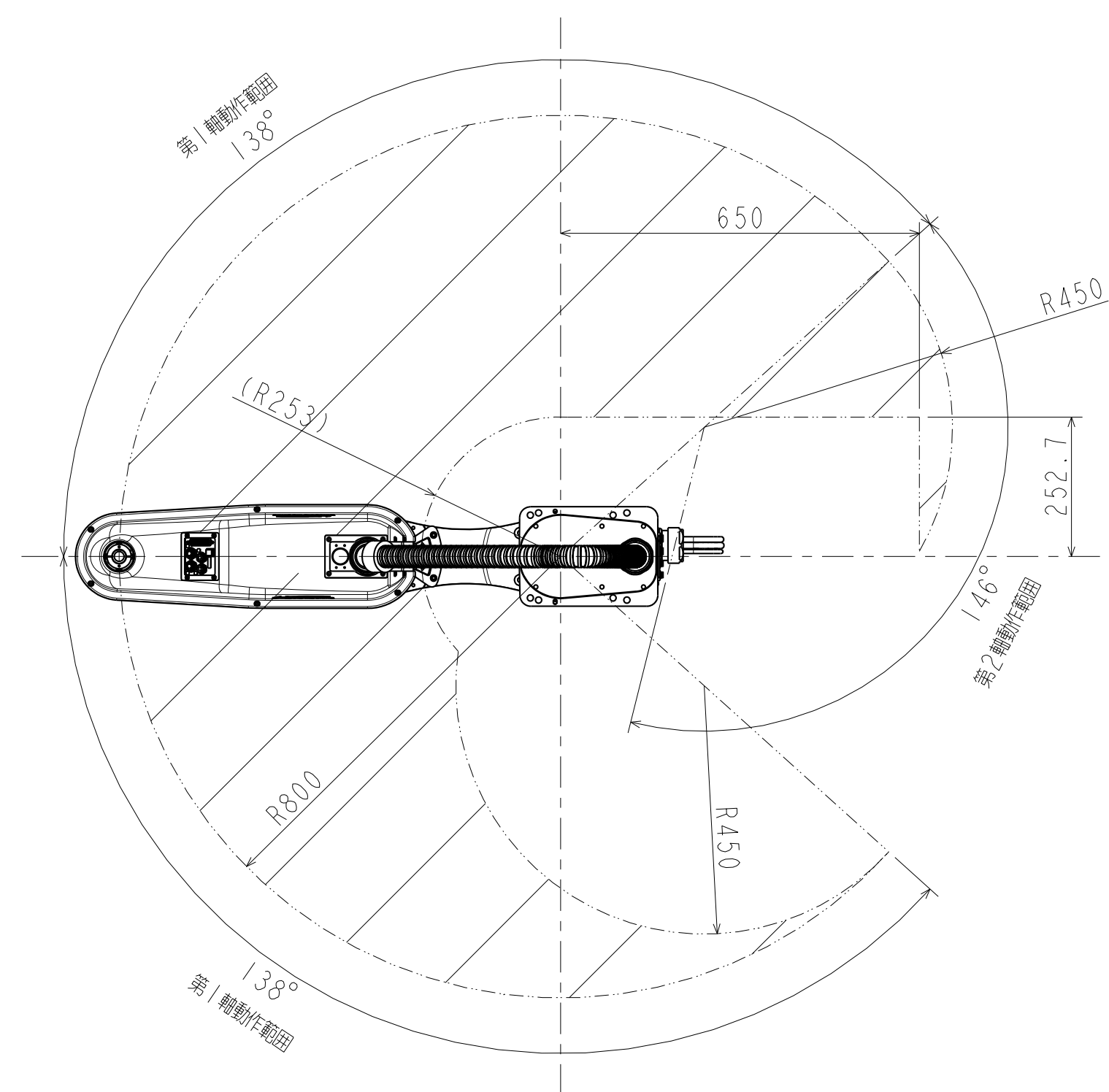
左手系動作範囲
