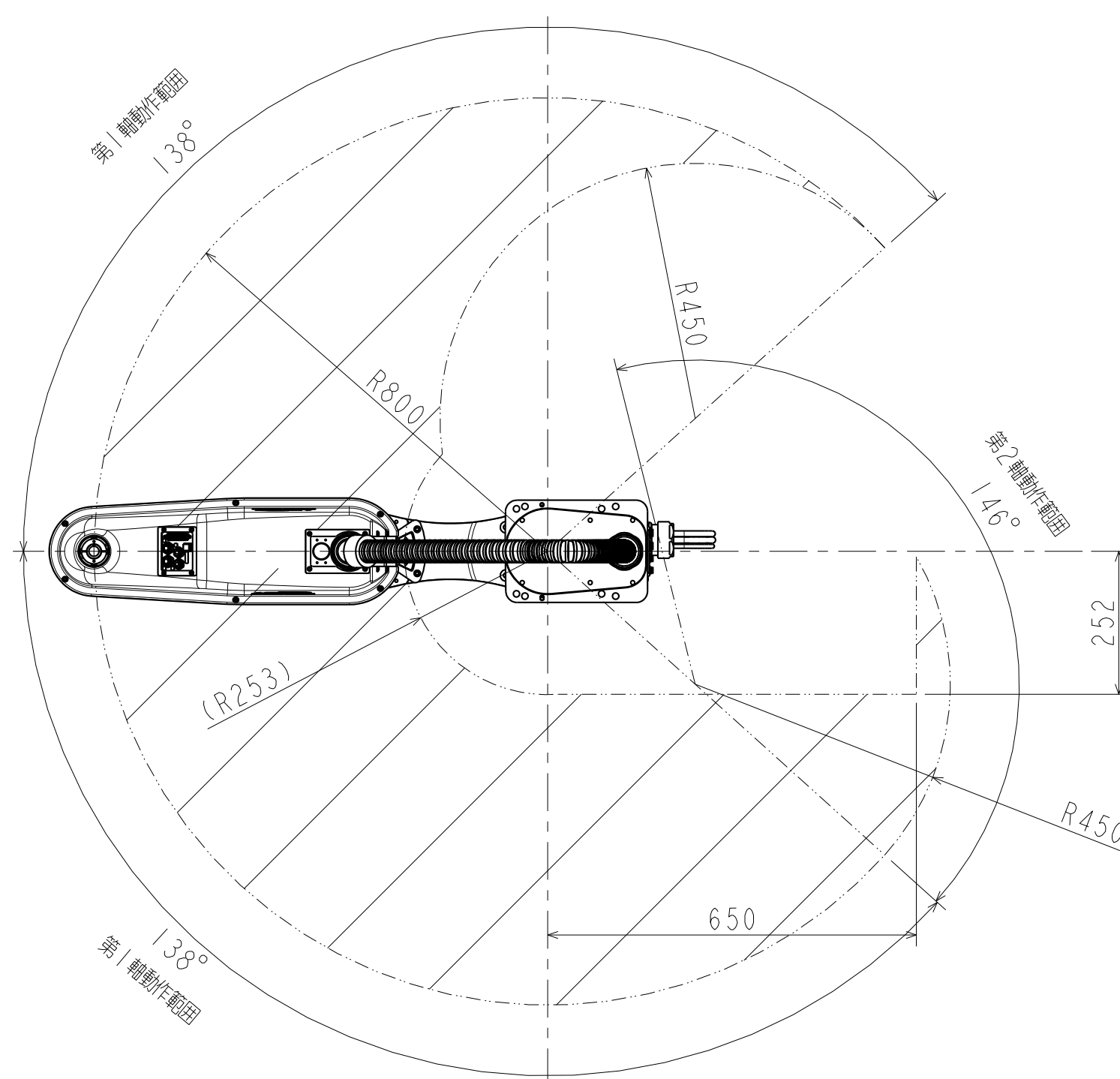
右手系動作範囲
