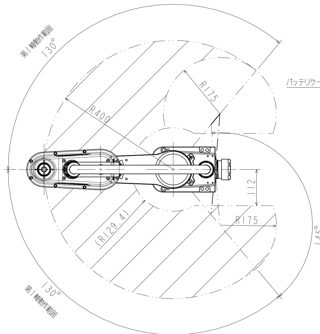
左手系動作範囲
