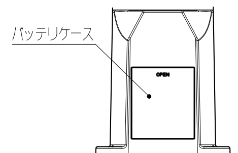
Z矢視
