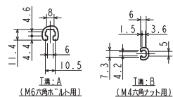
(M6六角ボルト用)
