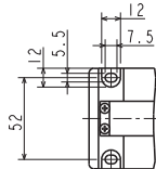
X軸長穴部詳細
