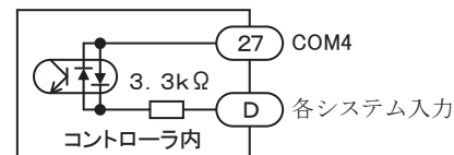
システム入力回路（NPN、PNP入力共通）
