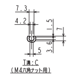
(M6六角ボルト用)
