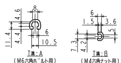
寸法: B (M4穴用ナット用)
