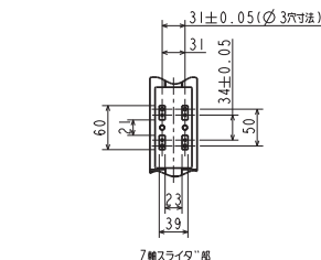
Z軸スライダ部
