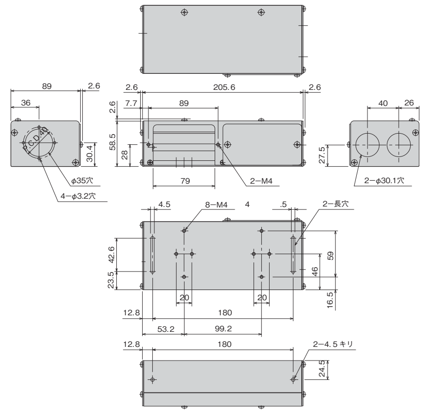
[BA10-BX-F20] フレキダクト (BA10-FD-□□□) 専用
