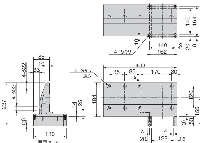
[BA1T7-BK-P06] 材質：アルミ合金 質量 0.5kg
