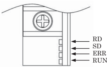
CC-Link 状態表示LED部
