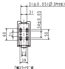
Z軸スライダ部
