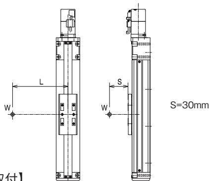
負荷形態Ⅴ【垂直取付】
