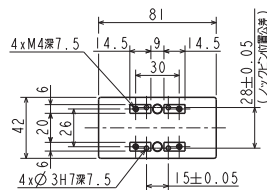
Y軸スライダ部詳細
