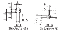
(M6六角ボルト用)
