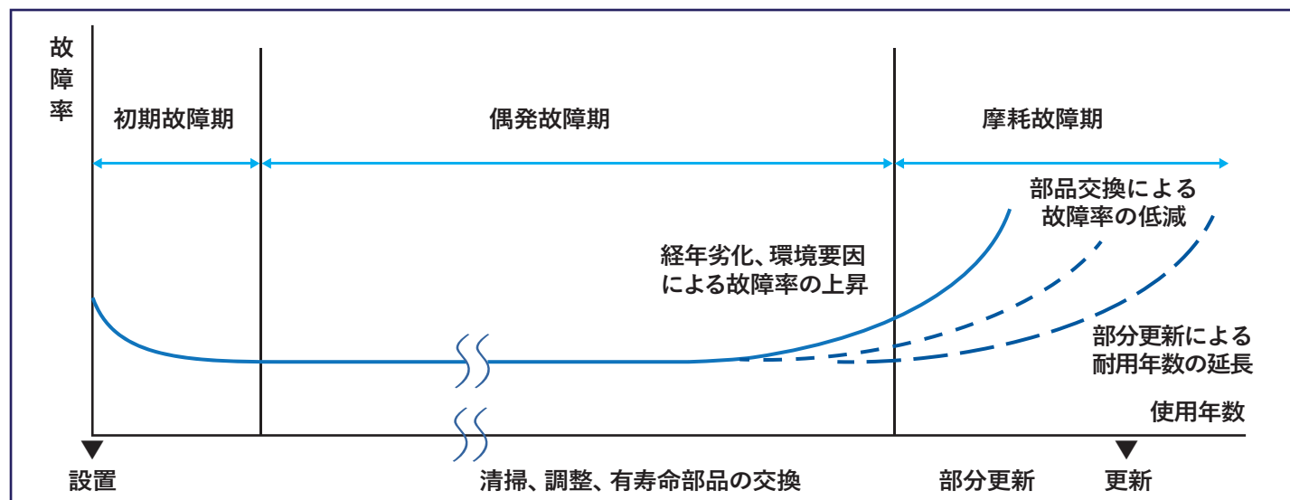
バスタブ曲線(故障率曲線) Failure rate curve
